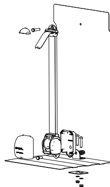
Exemple avec l'enrouleur installé sur le plancher du véhicule.
